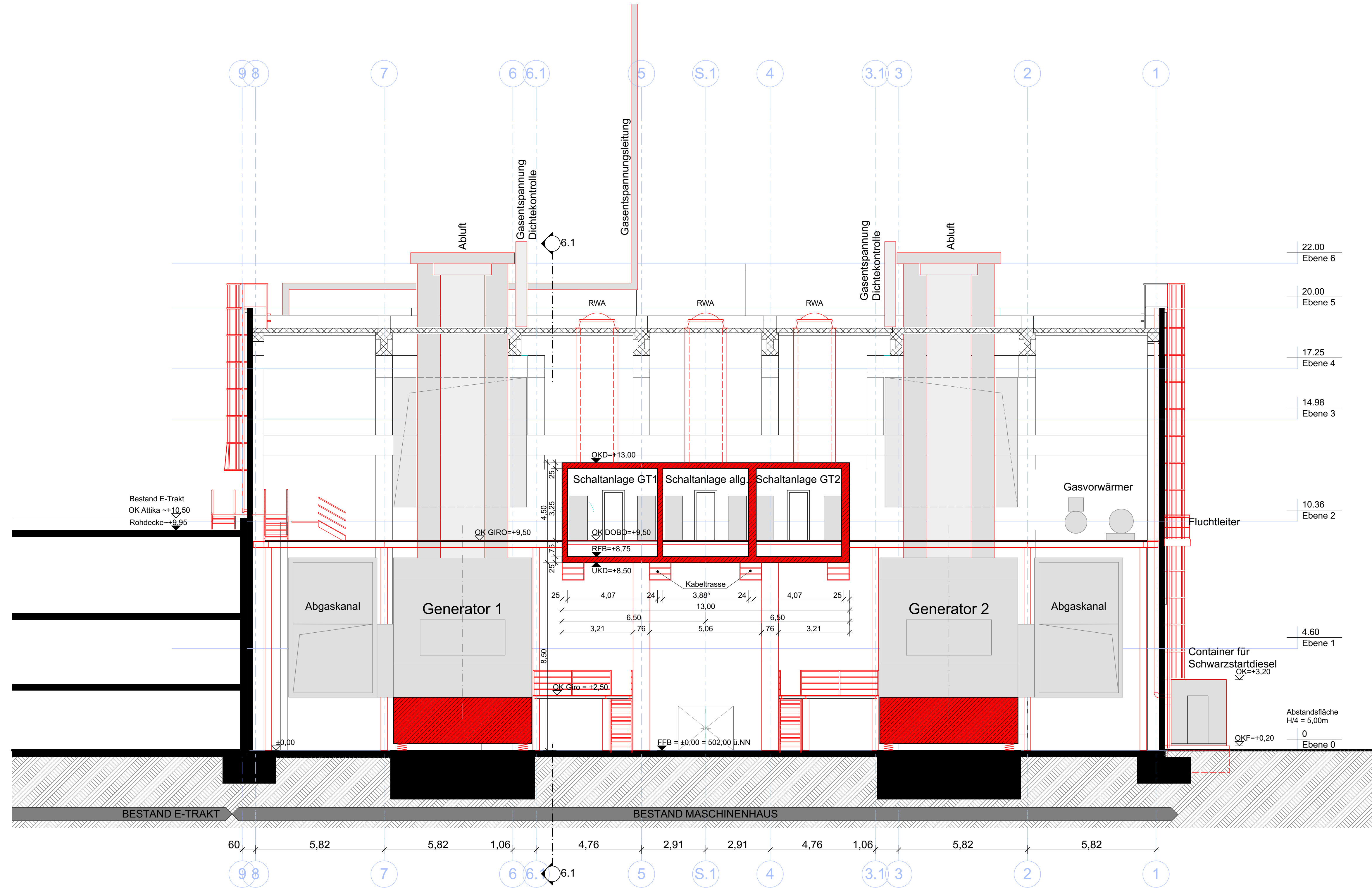
Schnitt Achse G.1 - Maschinenhaus
